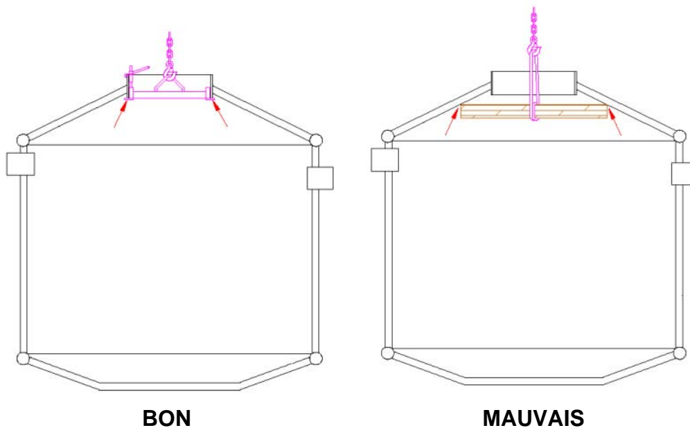
Figure 4 : levages correct et incorrect de la cuve BLUEVITA TORNADO
