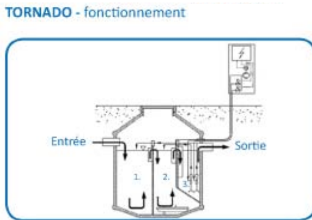
Figure 1 : Montage schématique d'une microstation TORNADO
