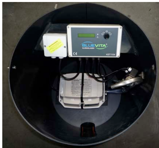
Figure 2 : Colonne de commande avec système de commande premium KST1104, surpresseur avec piston axial et 2 électrovannes
