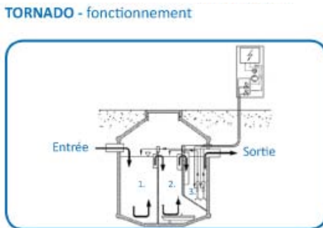
Figure 1 : Montage schématique d'une microstation BLUEVITA TORNADO
