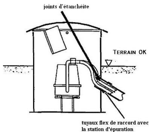
Figure 6 : Schéma d'installation de la colonne de contrôle externe
