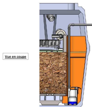
Figure B3 – Intégration de la pompe dans les modèles d'une filière de la Gamme « Filtre ECOFLO® Béton » sortie haute
