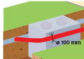
Détail du piquage de la ventilation secondaire, sur la canalisation de liaison entre fosse et filtre ECOFLO® Béton
