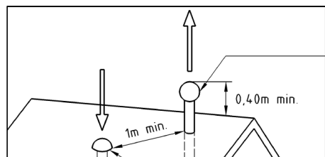
Implantation en faîtage et distance des ventilations
