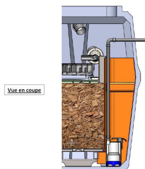
Figure A4 – Intégration du compartiment de relevage dans les filtres ECOFLO® Béton
