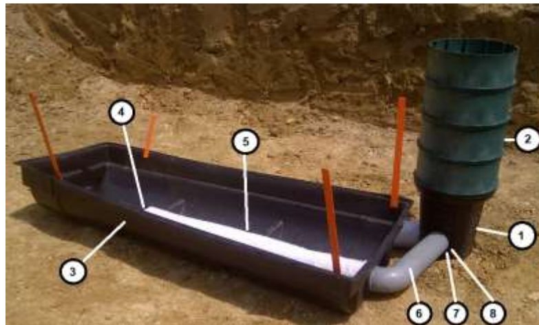
Figure 9 – Dispositif d'échantillonnage
