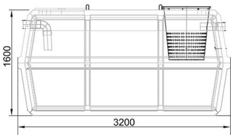
Exemple d'une cuve Gamma CLAIRFLO basse 7000
