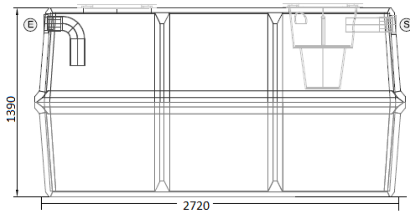
Exemple d'une cuve Gamma CLAIRFLO Basse 3000L
