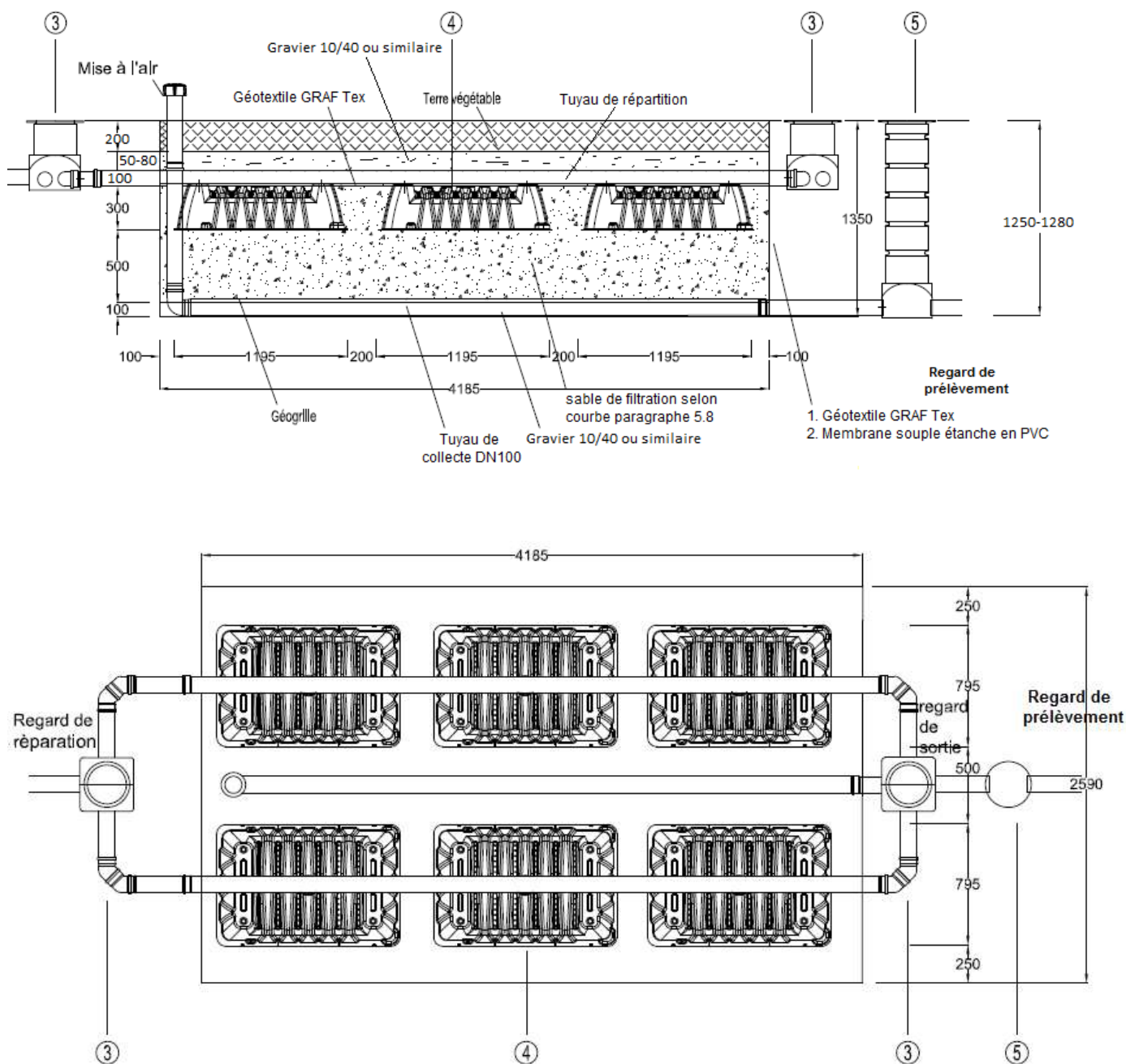
Exemple du Filtre Compact Biomatic 6 EH
