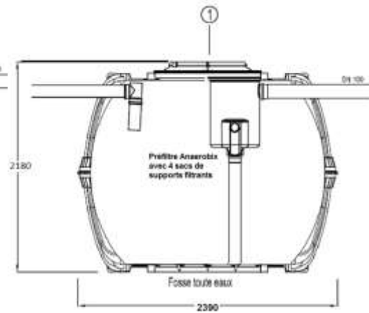
Exemple d'une cuve CARAT 6500 L
