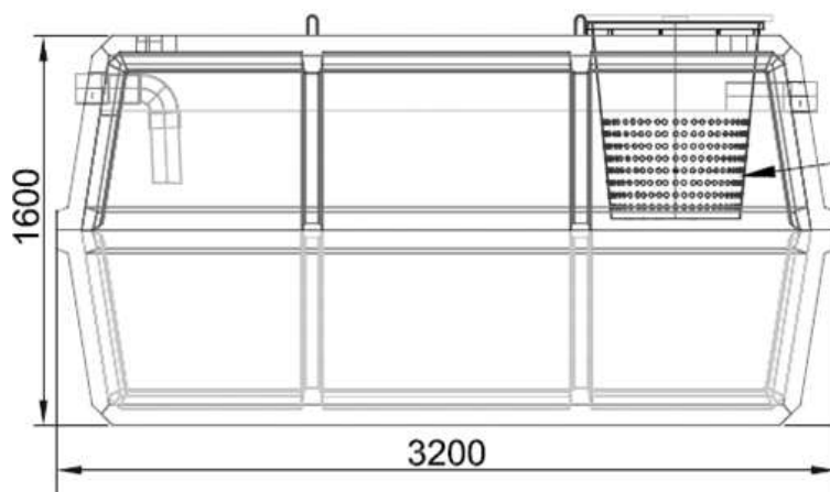
Exemple d'une cuve Gamma ULTRA 7000L
