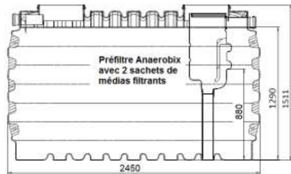
Exemple d'une cuve FTE 3000 L
