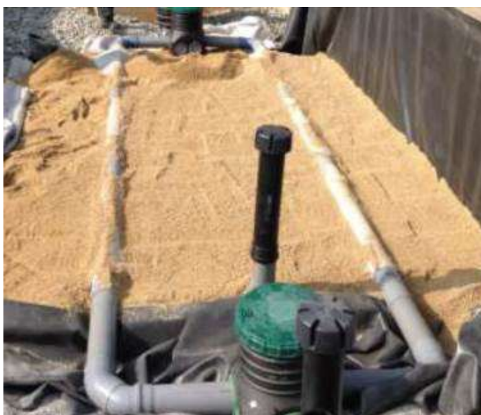
Exemple du Filtre Compact Biomatic 6 EH
