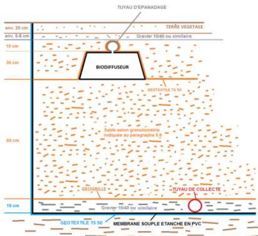
(Vue en coupe du filtre compact)
