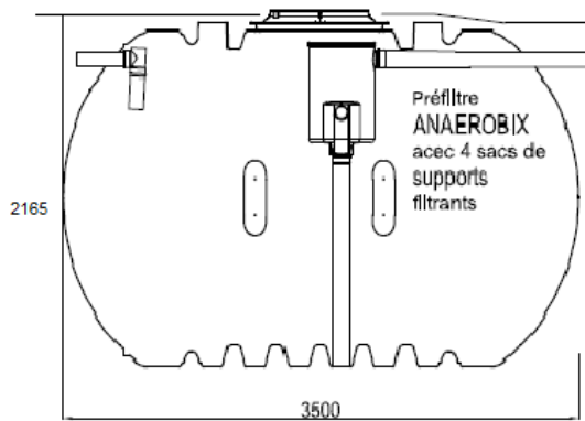
Exemple d'une cuve CARAT XL 8500 L
