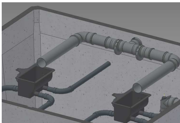
Fig-7 : Exemple de dispositif de répartition dans un filtre C-90 6,2m 3
