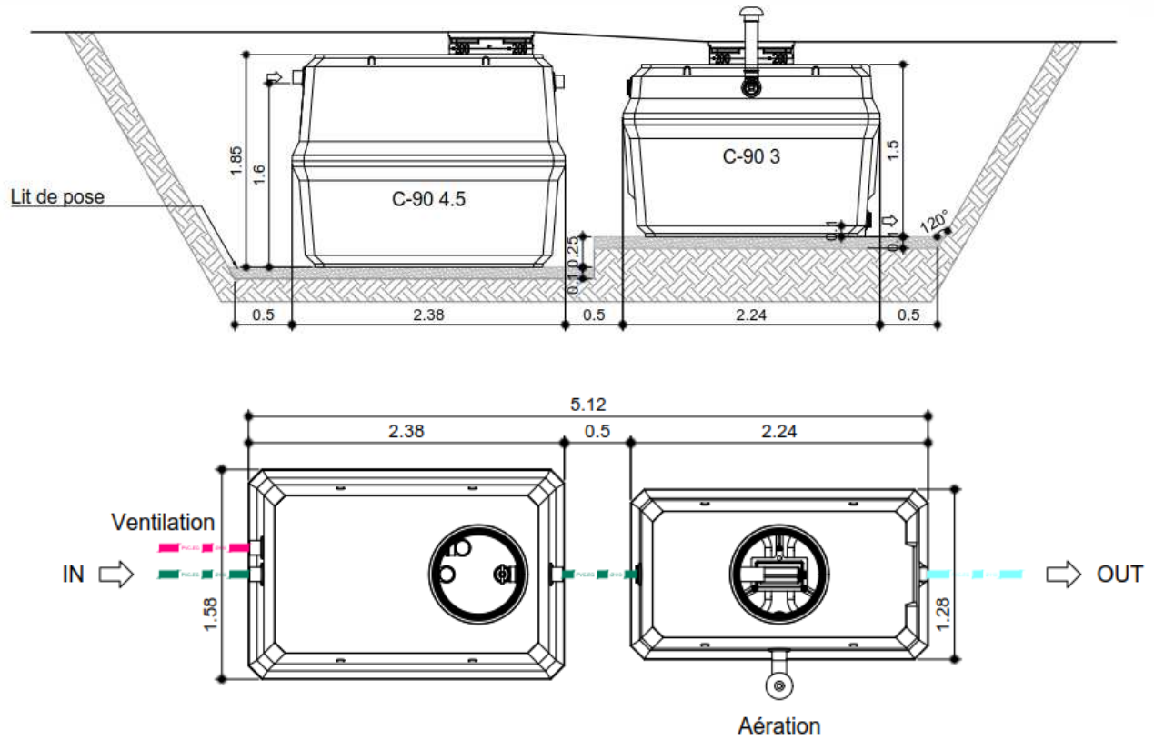
Fig-22 : X-Perco® France C-90 7EH Bicuve (4,5 m 3 )
