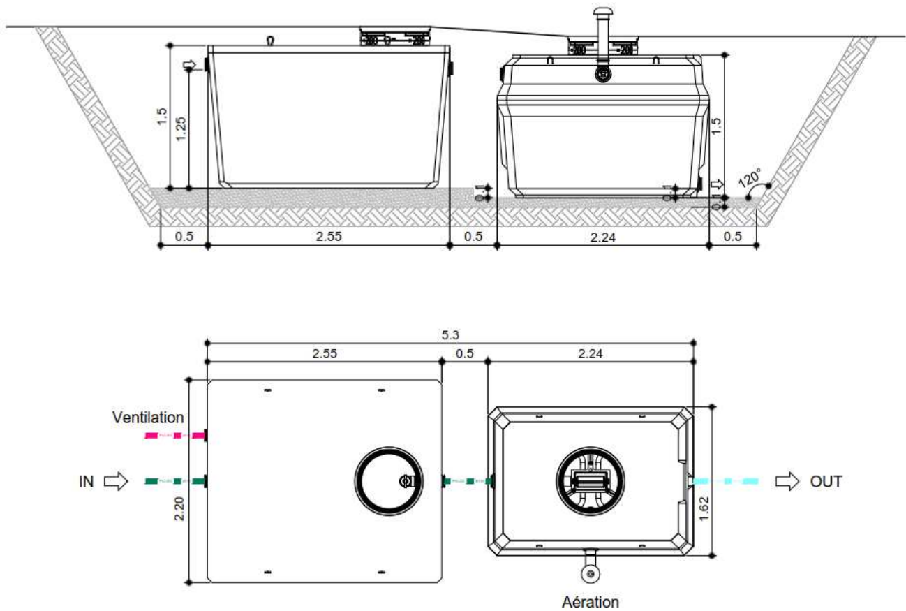
Fig-23: X-Perco® France C-90 10EH Bicuve (6,2 m 3 )
