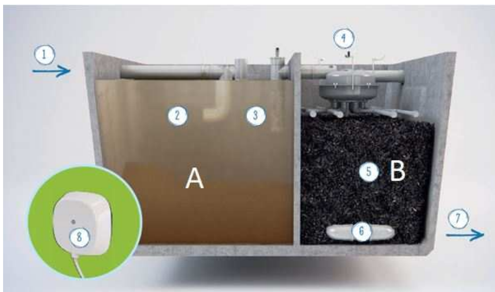
Fig-2 : Principe de fonctionnement de l'X-Perco® France C-90 5EH monocuve
