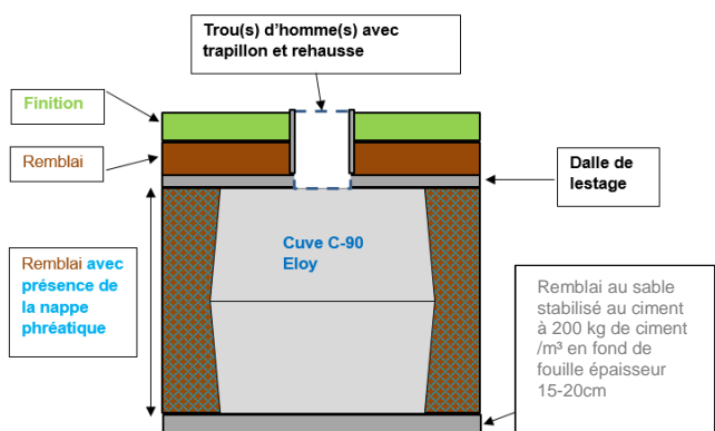
Fig-38 : Dalle de lestage
