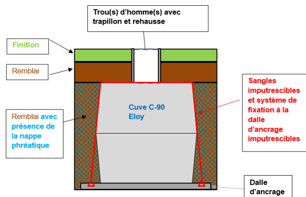
Fig-39 : Dalle d'ancrage
