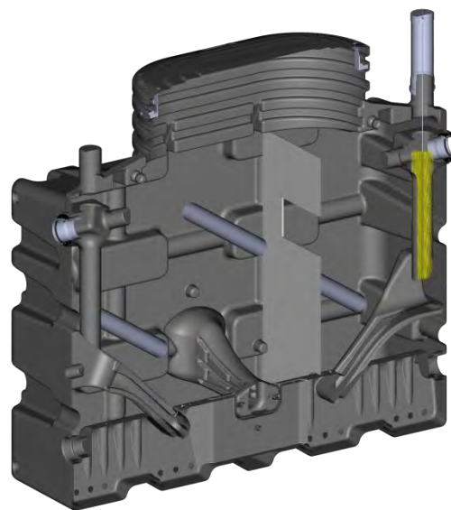
SCHEMA DE LA FOSSE TOUTES EAUX – Fig. 04
