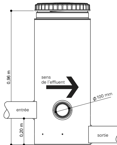
Boîte de prélèvement SP310P
