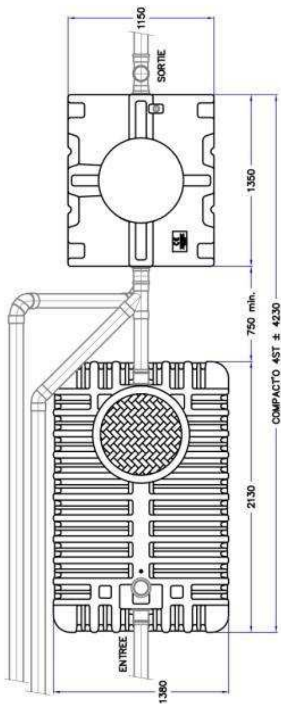
Fosse toutes eaux 3000 L
