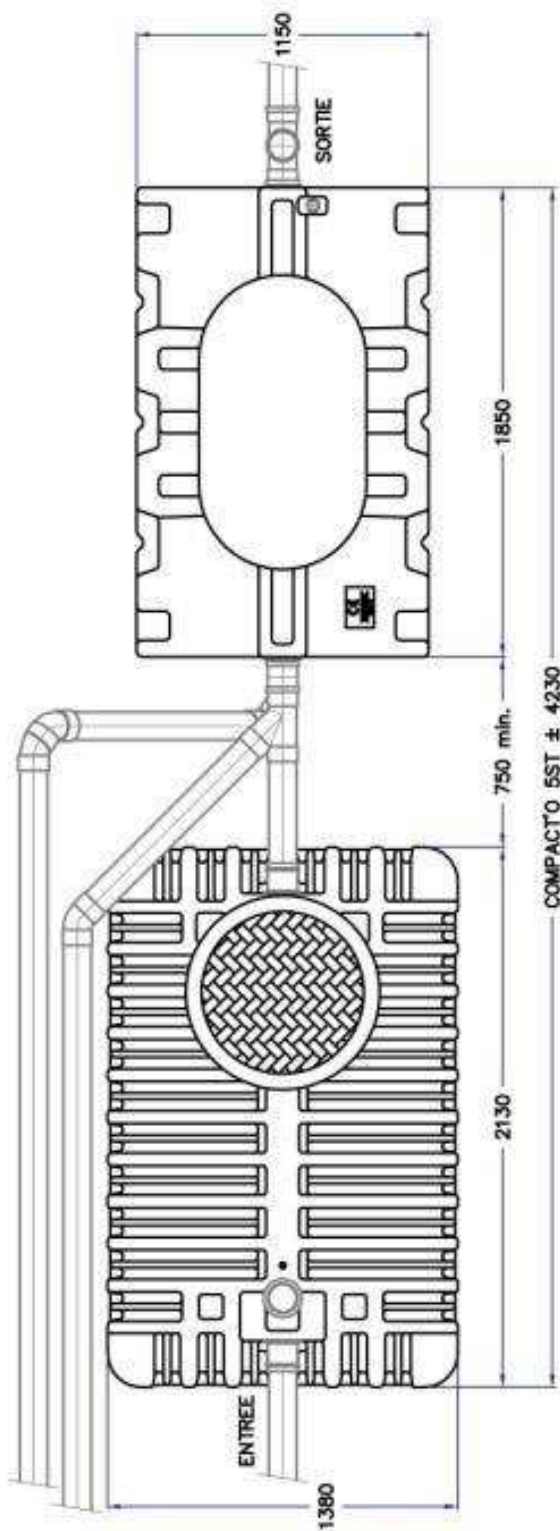
Fosse toutes eaux 3000 L
