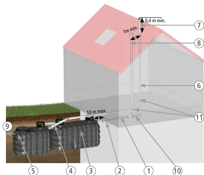
Schéma de raccordement de la ventilation haute pour une micro-station ACTIBLOC® LT 30-25 6EH posée en Ligne.
