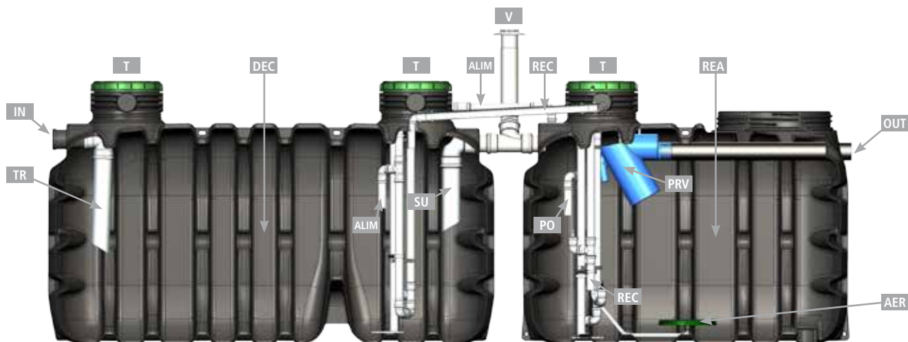
Vue de coupe d'une micro-station ACTIBLOC® LT 30-25 6EH posée en ligne.
