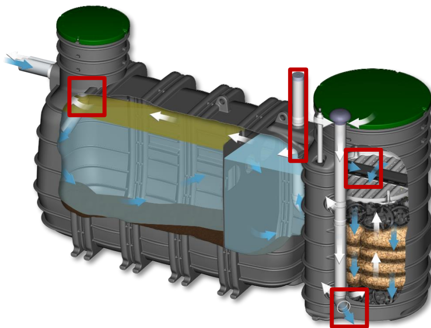
Points de contrôle pour vérifier l'écoulement des eaux sur une filière MONOBLOCK V3
