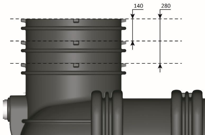
Niveau de découpe possibles des rehausses intégrées (exemple de la rehausse intégrée sur l'accès en DN 600 de l'unité de traitement primaire)
