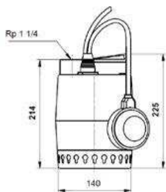
012K7700 UNILIFT KP250-A-1 50 Hz
