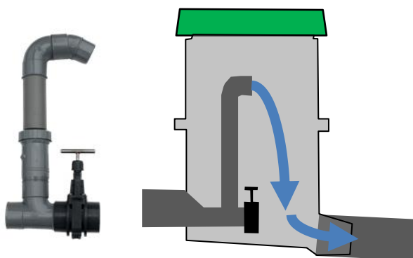
Dispositif de mise en charge du filtre à écoulement horizontal, posé à l'intérieur du regard de collecte permettant le prélèvement d'un échantillon
