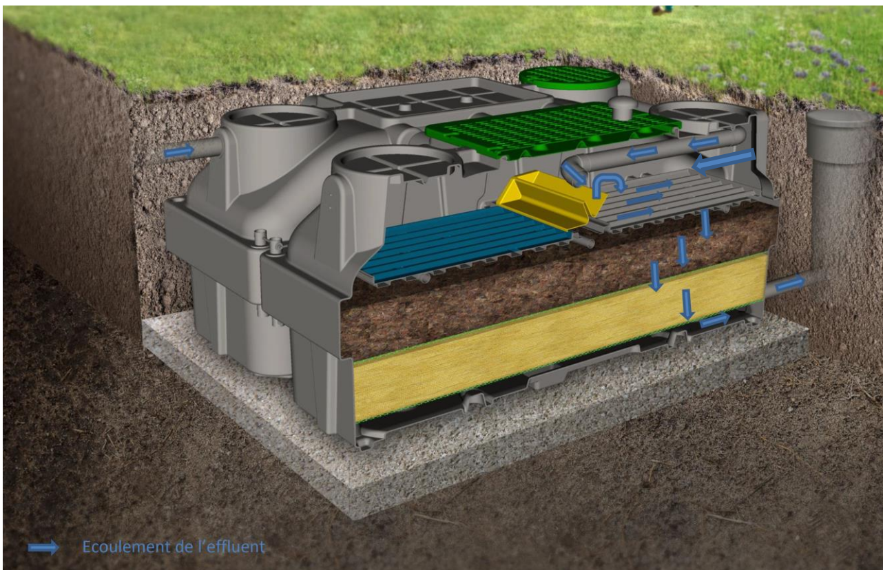
Figure 1 : Principe de fonctionnement des dispositifs STEPURFILTRE-FEA
